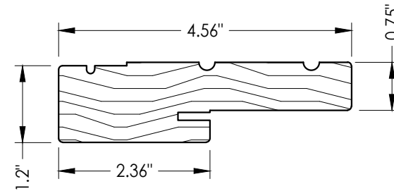
1 WOOD JAMB
